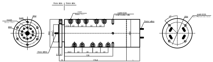
MAPH1040-01 Dimensions
