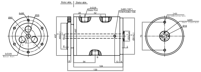
MQ300-04 Dimensions
