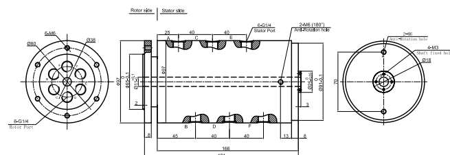
MQ600-03 Dimensions
